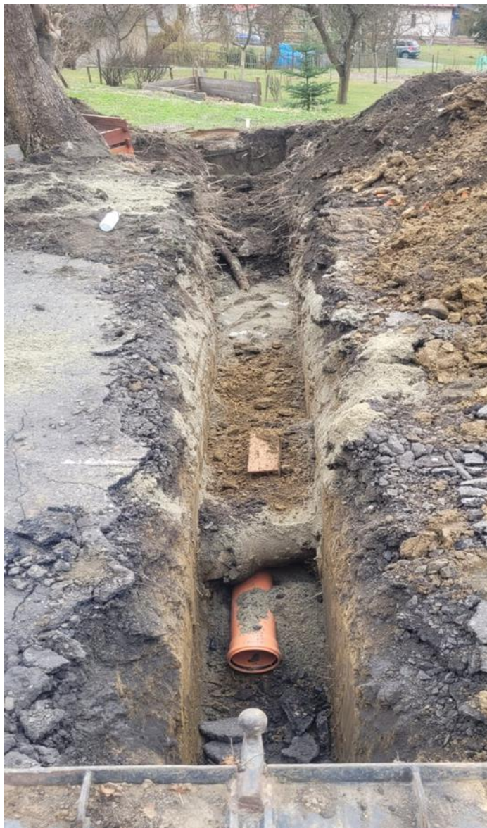
Zdjęcie 5 Wykop obrazujący wymianę sieci kanalizacyjnej w rejonie Istebnej Haratyki.
